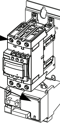
FIG. 2 : Reversing Starter Assembly / Ensamble de arrancador reversible / Assemblage du démarreur inverseur
