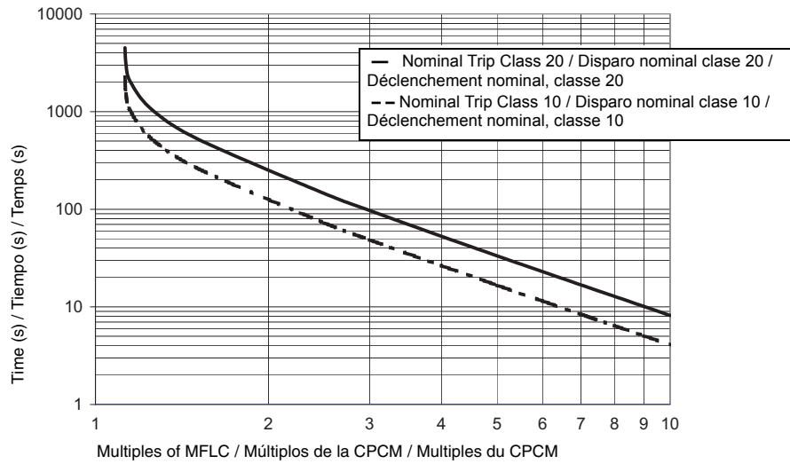
FIG. 7 : Trip Curves / Curvas de disparo / Courbes de déclenchement
