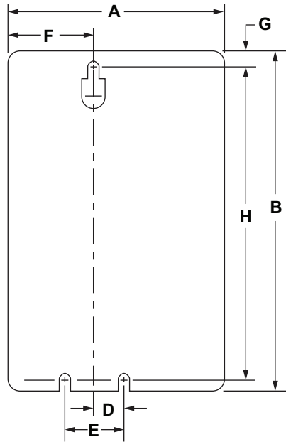
TABL. 2 : Baseplate Dimensions, in. (mm) / Dimensiones de la placa base, pulg (mm) / Dimensions du socle, po (mm)
