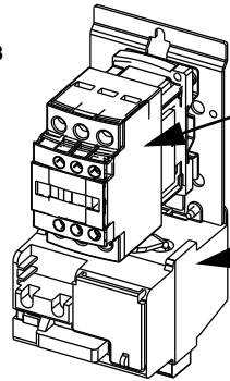
FIG. 2 : Reversing Starter Assembly / Ensamble de arrancador reversible / Assemblage du démarreur inverseur
