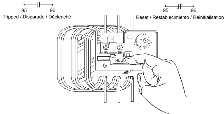
FIG. 6 : Resetting the SSOLR / Restablecimiento del RSES / Réinitialisation du RSCT
