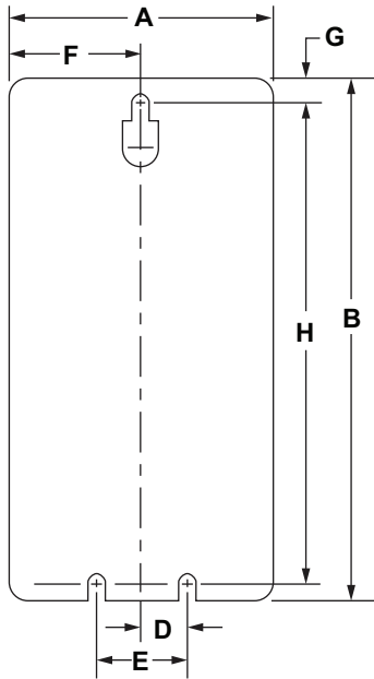
TABL. 2 : Baseplate Dimensions, in. (mm) / Dimensiones de la placa base, pulg (mm) / Dimensions du socle, po (mm)
